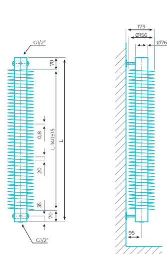
76x2,5x156 VERTIKAL
