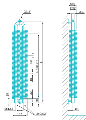
32x2x92 VERTIKAL
