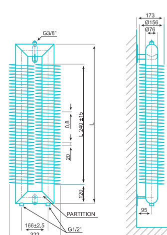
76x2,5x156 VERTIKAL
