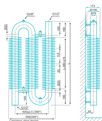
76x2,5x156 VERTIKAL VÄNSTER
