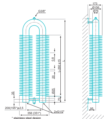
76x2,5x156 VERTIKAL
