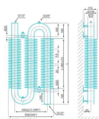
76x2,5x156 VERTIKAL HÖGER
