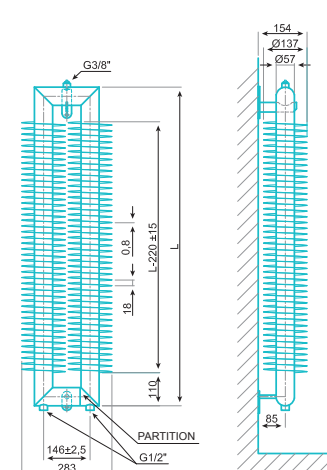
57x2,5x137 VERTIKAL
