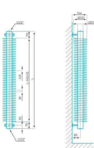
57x2,5x137 VERTIKAL
