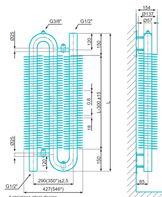
57x2,5x137 VERTIKAL VÄNSTER
